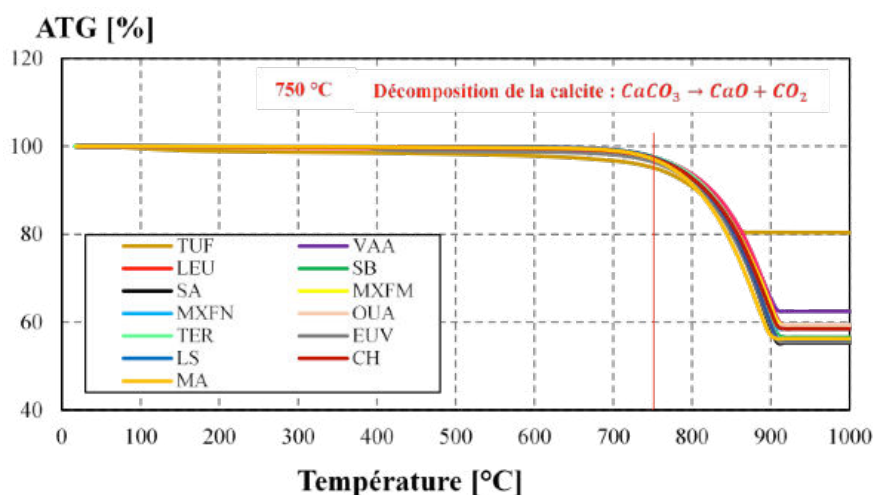
Figure 3 : courbes ATG - évolution de la perte de masse des 13 pierres calcaires de l'étude en fonction d'une élévation de la température
