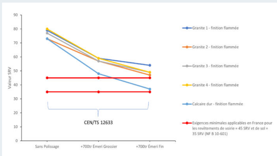
Valeur moyenne de glissance (SRV Humide) en fonction du polissage selon la norme CEN TS 12633 pour les différents granites et le calcaire dur en finition flammée
