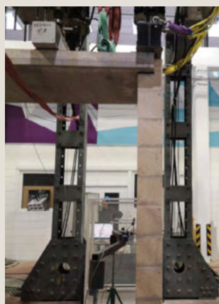
Réalisation de l'essai : chargement mécanique du mur de rive jusqu'à rupture Photo : CTMNC
