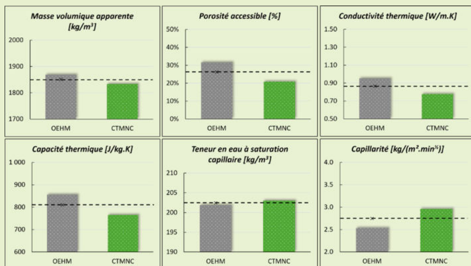
Comparaison de résultats de caractérisation, OEHM (Equipe DMS) et CTMNC, pierre de Vers-Pont-du-Gard.
