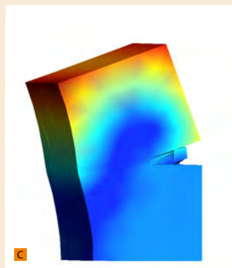
Résistance d'un trumeau à une sollicitation de compression excentrée de e_{mur}/6 , à température ambiante : (a) Maquette testée, (b) Mécanisme de rupture observé par corrélation d'images, (c) Mécanisme de rupture obtenu par l'approche cinématique numérique du calcul à la rupture (droits d'images : Elodie Donval, Thèse de doctorat)
