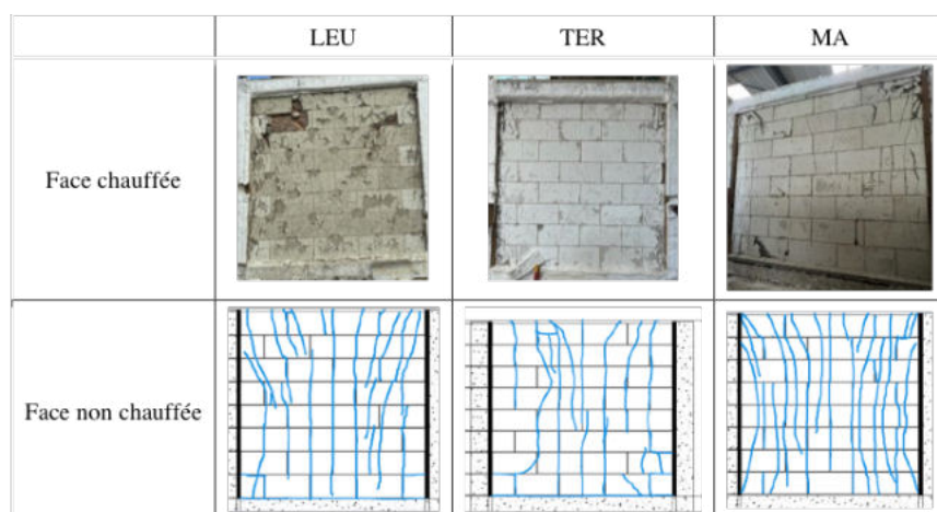
Figure 5 : fissures observées sur les faces chauffées et non chauffées des différents murs chargés
