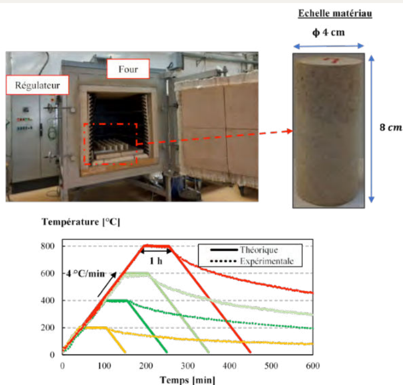
Figure 1 : four électrique Isartel-900 °C utilisé pour le chauffage des éprouvettes cylindriques (longueur 8 cm et diamètre 4 cm) à différents cycles de chauffage-refroidissement : 200, 400, 600 et 800 °C
