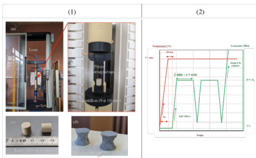
Figure 4 : dispositif des essais mécaniques à chaud disponible au CTMNC ; presse Zwick/Roell couplé à un four Maytec (1) ; programme thermo-mécanique de l'essai dit à chaud : phase initiale d'élévation de la température, suivie d'une phase de maintien de la température cible puis démarrage du chargement mécanique (2)
