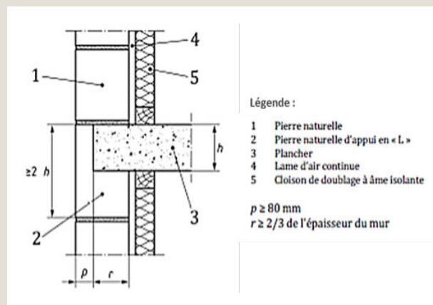
Schéma de la configuration d'un mur de rive, maçonné en pierre naturelle, supportant le plancher béton en appui partiel (extrait du NF DTU 20.1)
