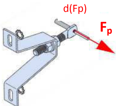
Figure A.2 : Vue en 3D d'un essai de chargement d'une attache de fixation dans la direction parallèle au support (détermination de d(F_p) )
