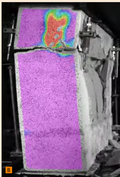
Résistance d'un trumeau à une sollicitation de compression excentrée de e_{mur}/6 , à température ambiante : (a) Maquette testée, (b) Mécanisme de rupture observé par corrélation d'images, (c) Mécanisme de rupture obtenu par l'approche cinématique numérique du calcul à la rupture (droits d'images : Elodie Donval, Thèse de doctorat)
